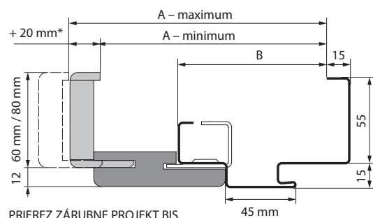
PRIEREZ ZÁRUBNE PROJEKT BIS
