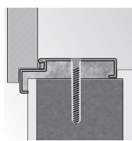
rohová zárubňa veľká montáž pomocou príchytiek
