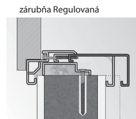
zárubňa Regulovalná
