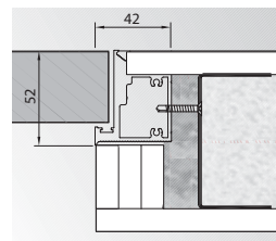
bezfalcové (otváranie von)
