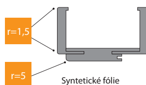
Syntetické fólie
